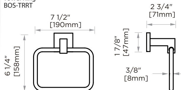
Towel Ring BOS-TRRT
