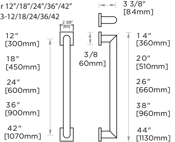
Grab Bar 12"/18"/24"/36"/42" SYD-GB5-12/18/24/36/42
