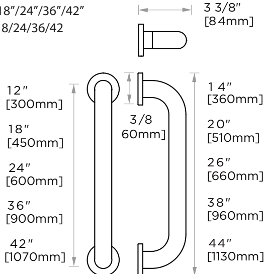
Grab Bar 12"/18"/24"/36"/42" SYD-GB5-12/18/24/36/42
