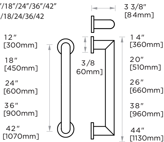
Grab Bar 12"/18"/24"/36"/42" SYD-GB3-12/18/24/36/42
